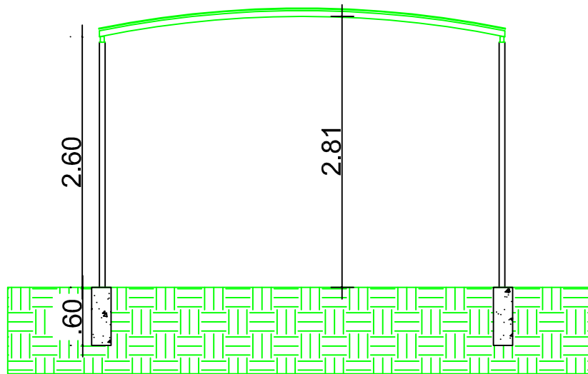
02 Corte BB'
