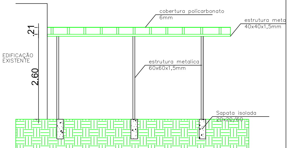
01 Corte AA'
