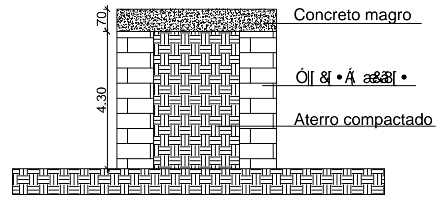
Detalhe banco 02
