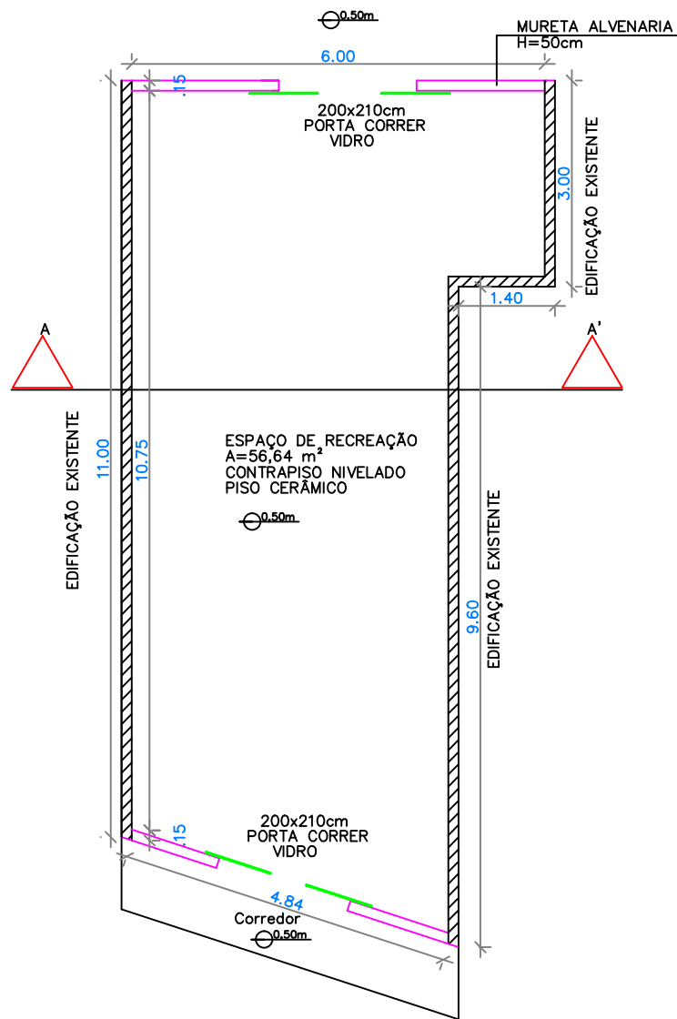
01 Planta Baixa A=58,27m 2
