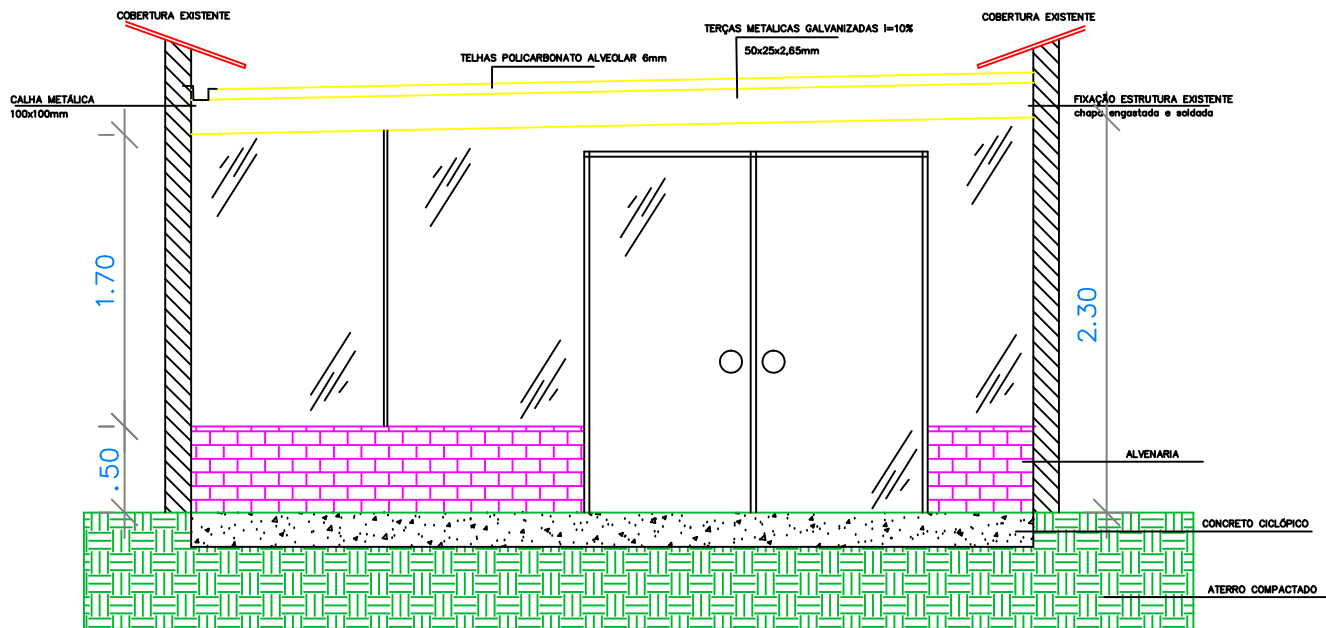
01 Corte AA'
