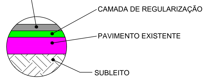
DETALHE 1 SEM ESCALA
