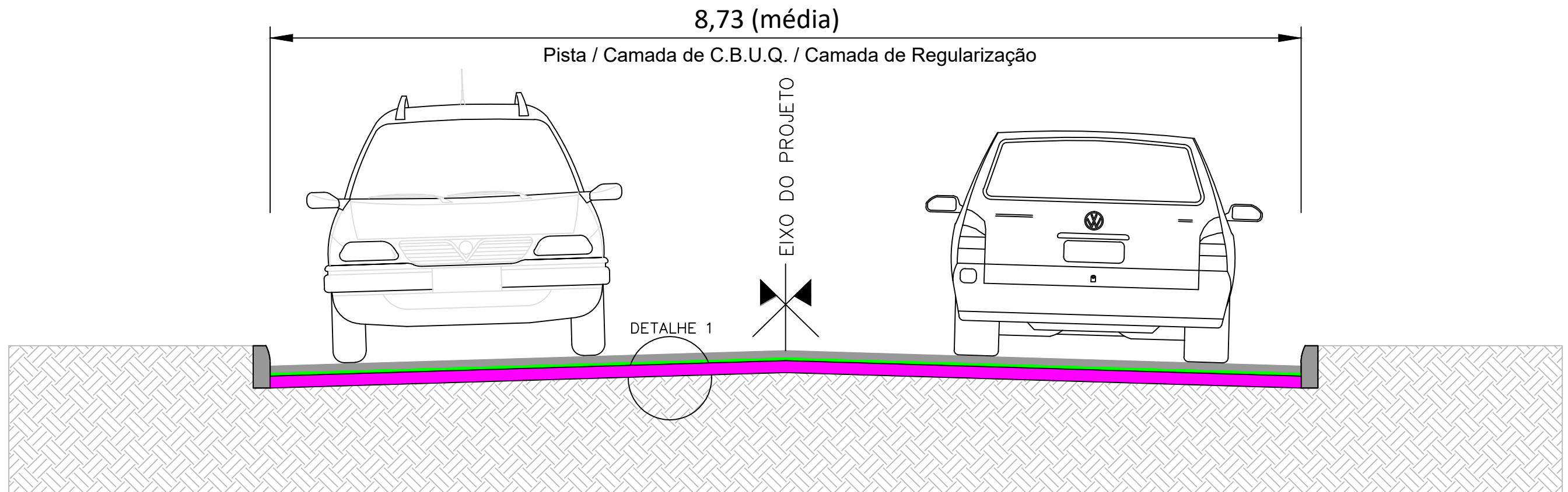
SEÇÃO TIPO DE PAVIMENTAÇÃO SEM ESCALA
