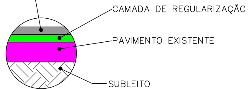
DETALHE 1 SEM ESCALA
