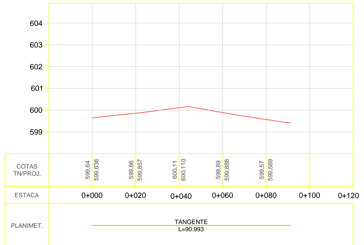
PERFIL Rua Riachuelo T2
