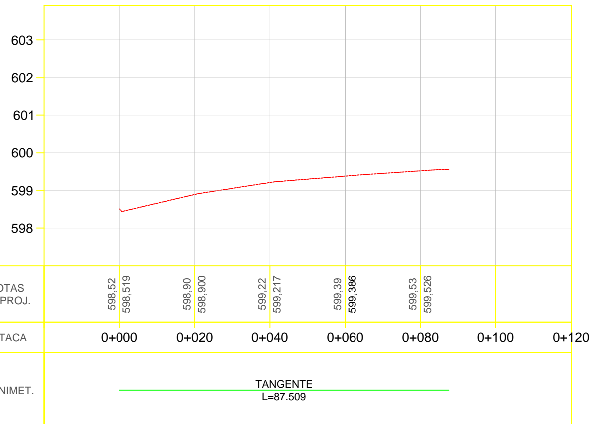
PERFIL Rua Riachuelo T1
