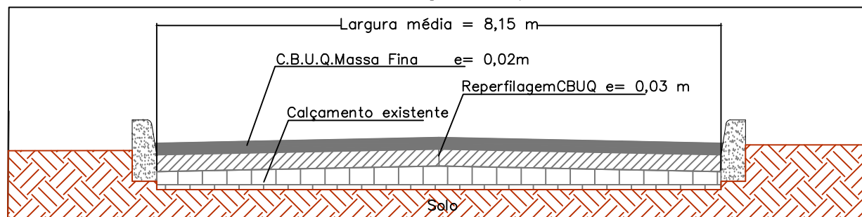
Seção Tipo
