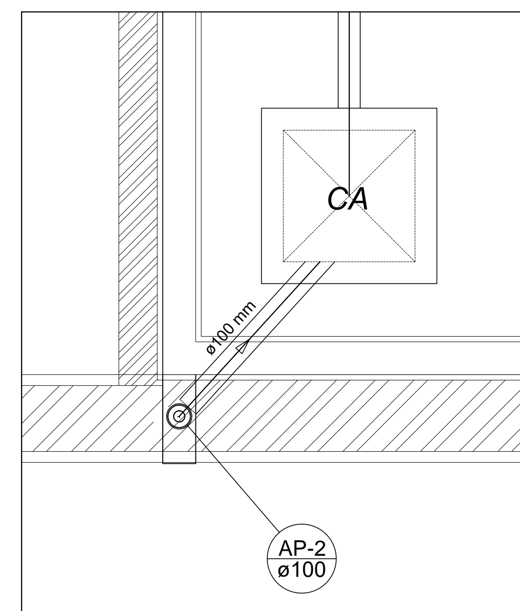
Detalhe S1 escala 1:20
