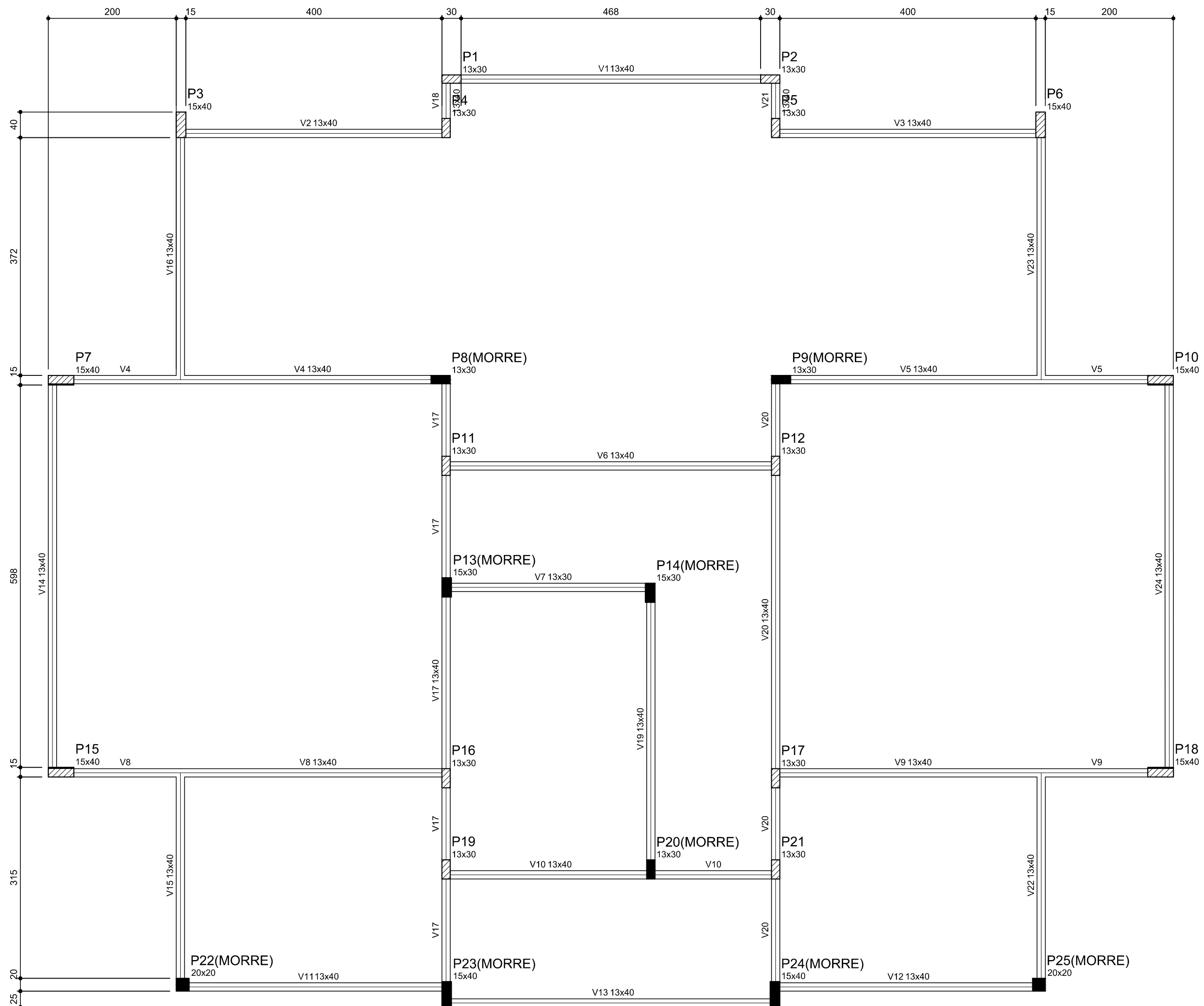
Forma do pavimento Nivel 000 escala 1:50
