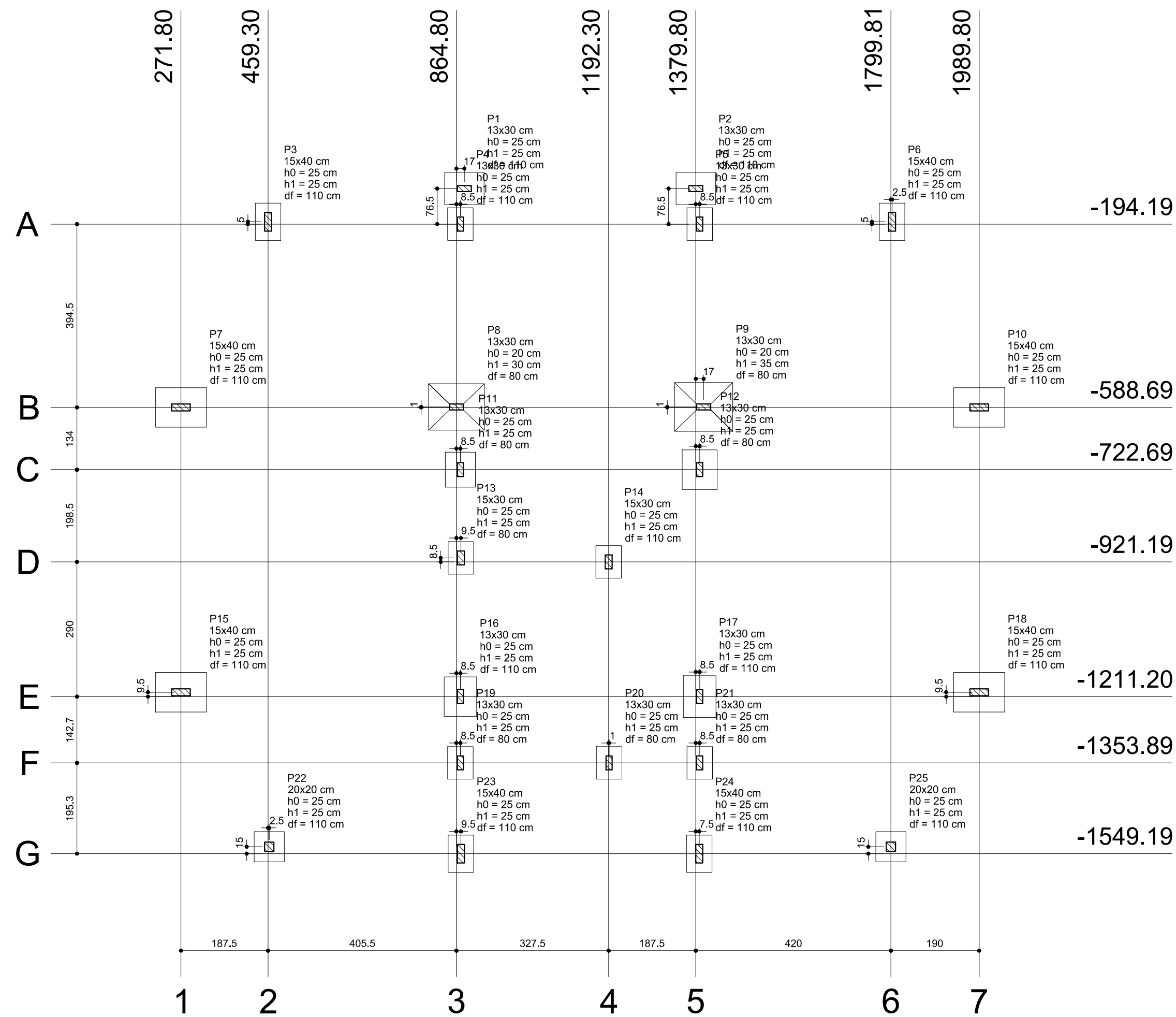
Planta de locação escala 1:75
