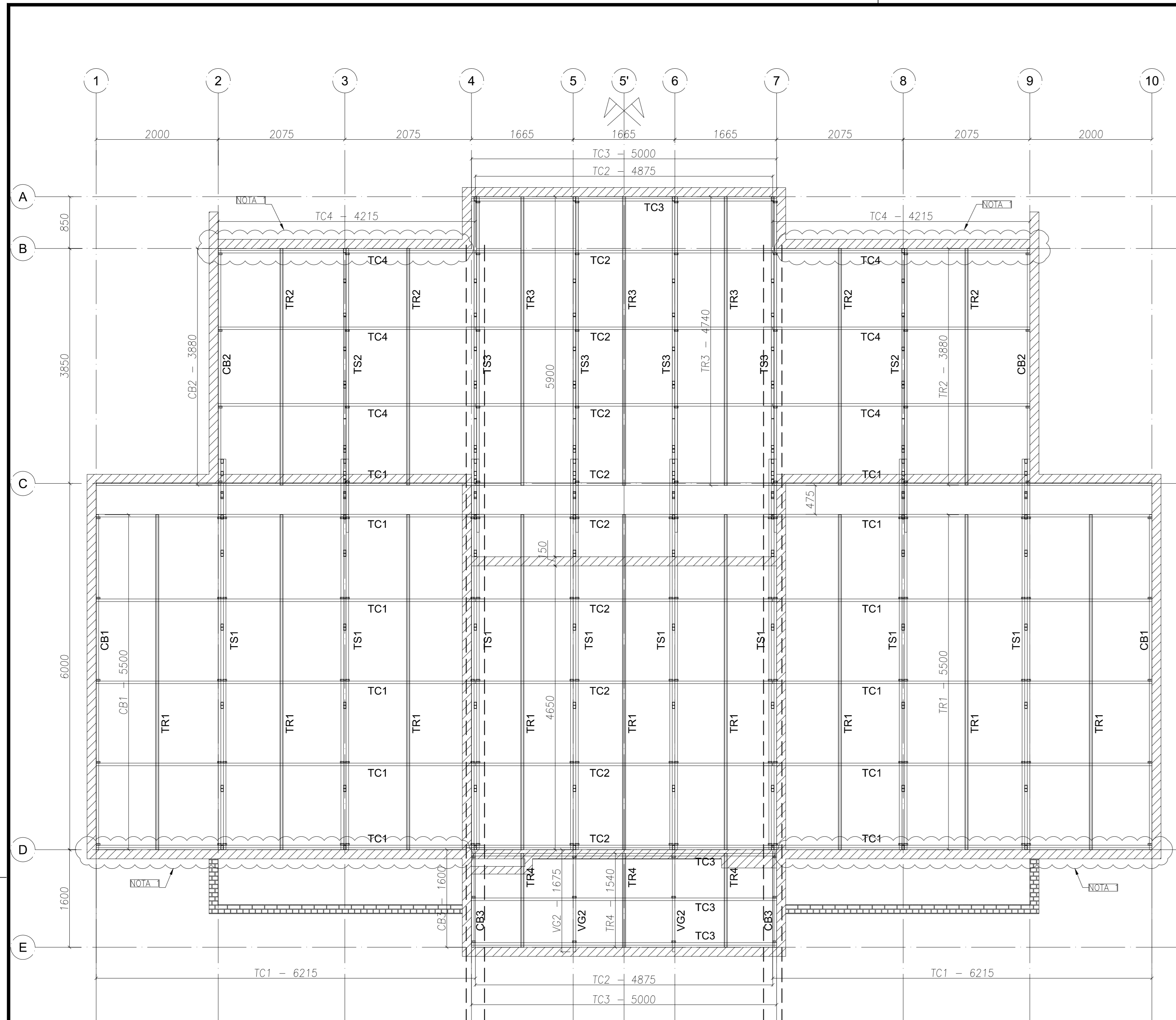
PLANTA DE COBERTURA - CAIBROS, TRELIÇAS, TERÇAS, TRAVAMENTOS e LUVAS Escala 1 : 5 0
