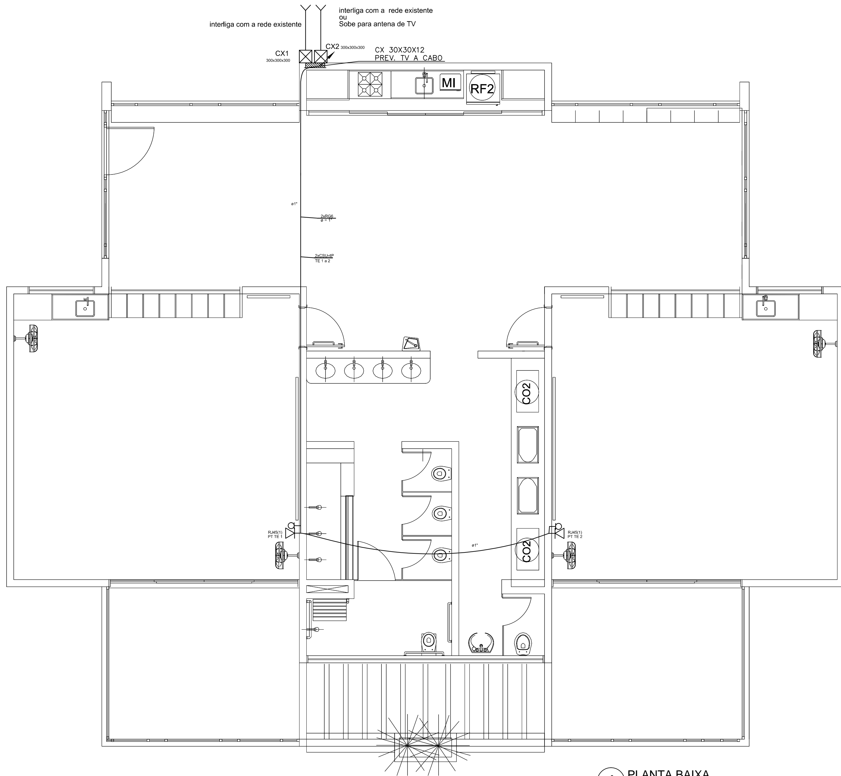
1 PLANTA BAIXA ESCALA 1/50
