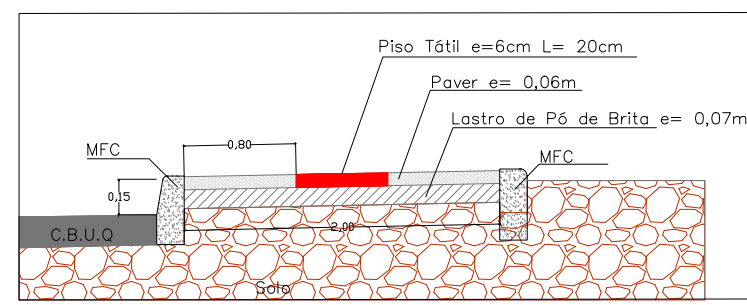
Corte Passeio
